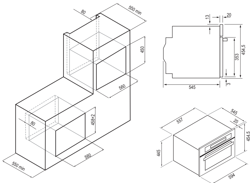
Схема встраивания духового шкафа.
