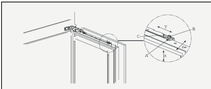
13-сурет: Шкаф есігінің жоғарғы қапталын реттеу
