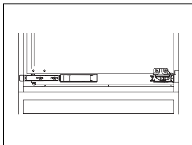
Установка нижнего крепежного узла
