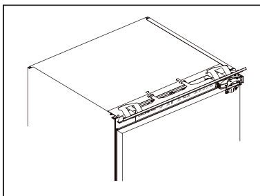
Установка верхней прокладки
